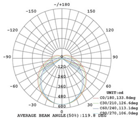
E-B20W-CC | 4000K
