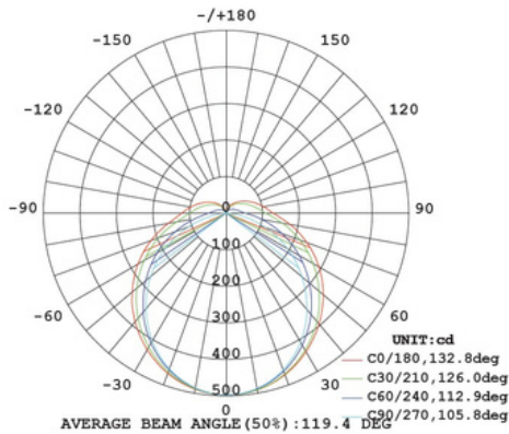
E-B20W-CC | 3000K
