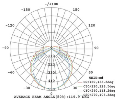
E-B20W-CC | 5700K
