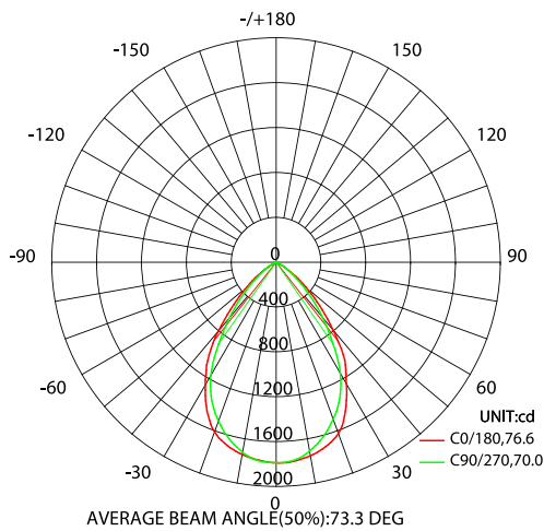
SL32W-CC | 3000K
