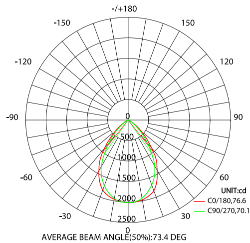
SL32W-CC | 4000K
