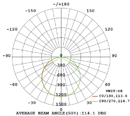
BLP36W-120/30 | 5700K
