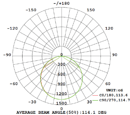
BLP36W-120/30 | 4000K
