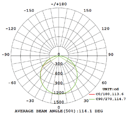
BLP36W-120/30 | 3000K
