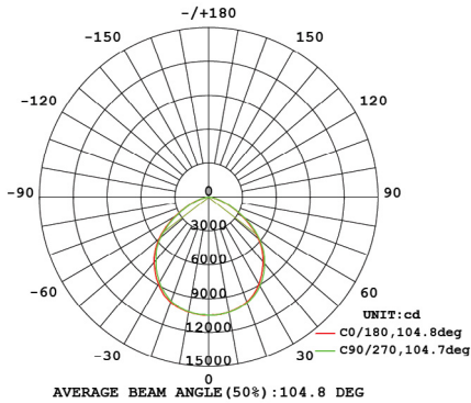
UFO-200W-E | 6000K
