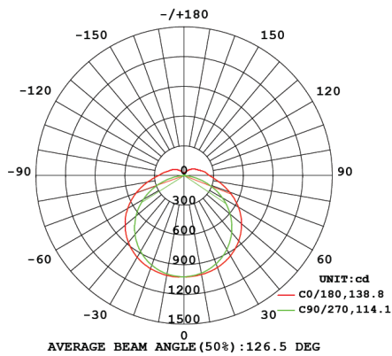
WBB-38W-CC | 5700K
