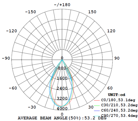
TL30W | 4000K
