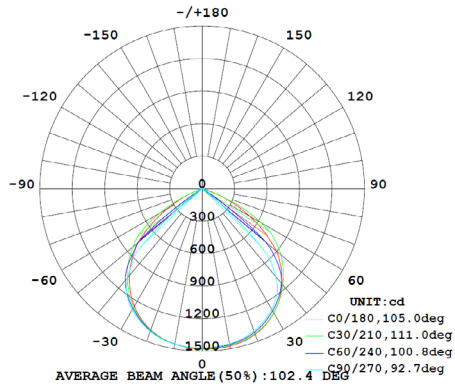
LED-SL35W-NW | 4000K
