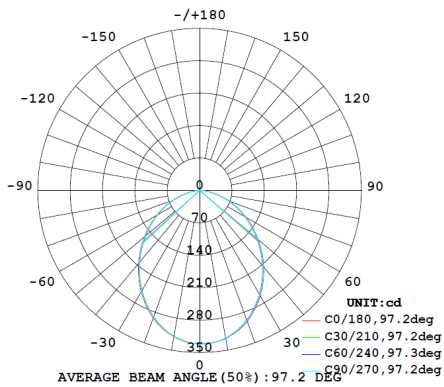
ID8W-CC-F | 5700K
