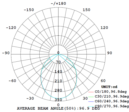
ID8W-CC-F | 3000K
