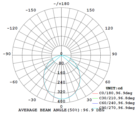
ID8W-CC-F | 4000K
