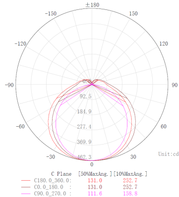
B20W-CC-MS | 6000K
