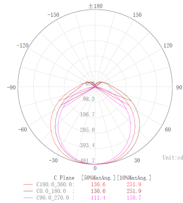
B20W-CC-MS | 4000K
