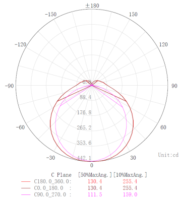
B20W-CC-MS | 3000K
